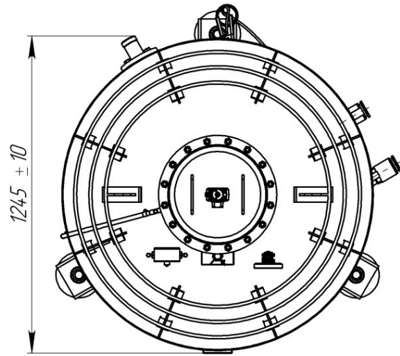
Рисунок А3.а Габаритные и присоединительные размеры установок УПМ СГ 500 и УПМ СГ 1000 модификации МВТ
