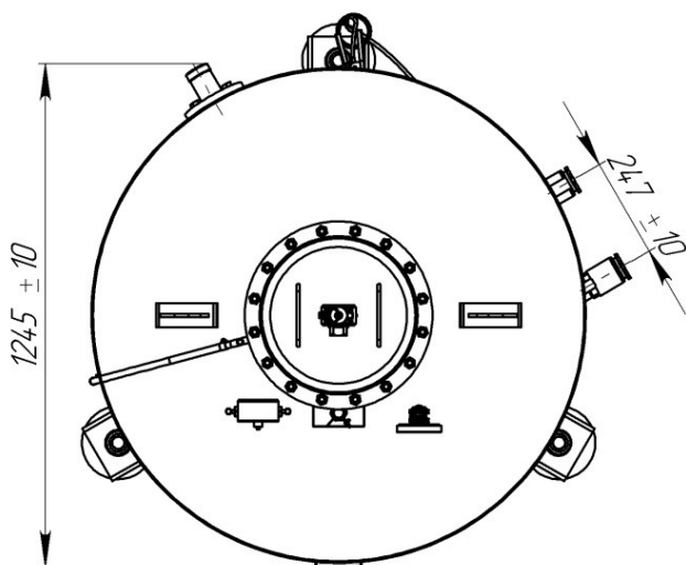
Рисунок А.3 Габаритные и присоединительные размеры установок УПМ СГ 500 и УПМ СГ 1000 модификации М
